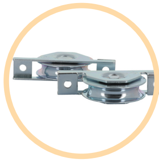
Galet Acier Galvanisé sur roulement à bille étanche diamètre 80mm livré monté sur le portail
